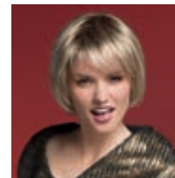
VISTA ** page 21
